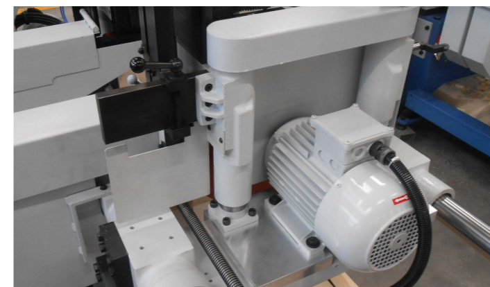
EJEMPLO UNIDAD DE CORTE
